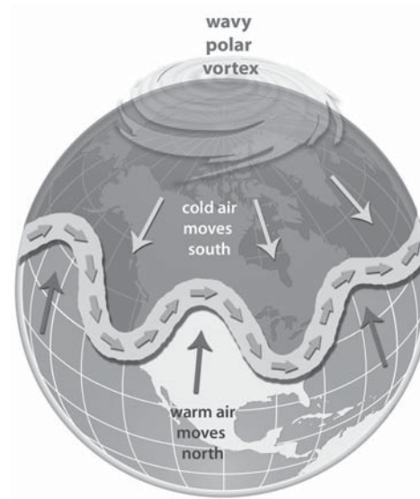
Bei einem schwachen Polarwirbel bilden die Höhenwinde Wellen, wodurch die kalte Luft sich nach Süden bewegen kann.
