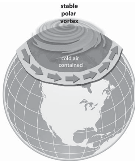
Ein stabiler Polarwirbel hält die kalte Luft im hohen Norden fest.
